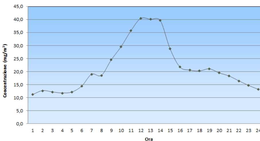
SITO RICETTIVO "TIRRENO POWER" - DAL 01/08/2017 AL 11/09/2017 Polveri frazione PM10: giorno tipo
