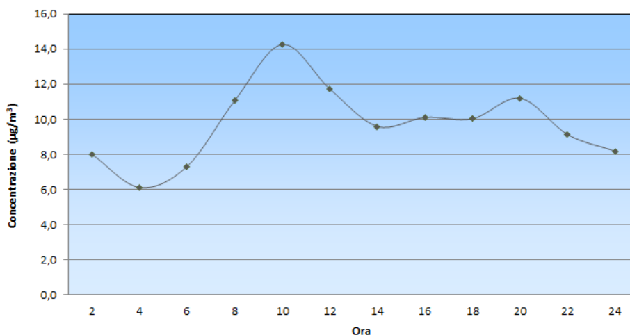
SITO RICETTIVO "SANTA RITA" - DAL 13/07/2017 AL 18/08/2017 Polveri frazione PM10: giorno tipo
